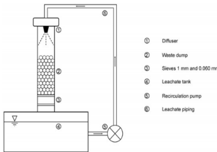
Figura 7 Proceso de lixiviación para la recuperación de cobre
