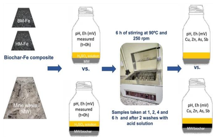
Figura 4 Recuperación potencial de zinc a partir de un residuo minero
