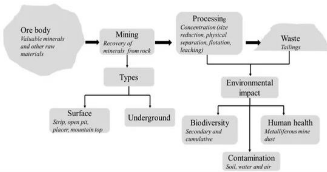
Figura 5 Procedimiento de recuperación de metales
